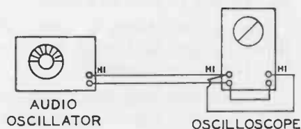
FIG. 2 PHASE INDICATOR
